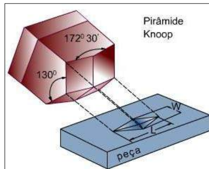
Figura 9. Penetrador Knoop
