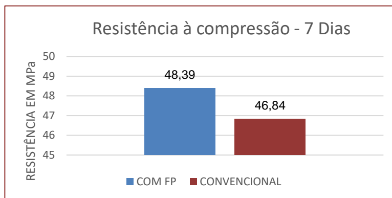
Figura 3: Resistência à compressão média do concreto com fibra e sem fibra com idade de 7 dias.
