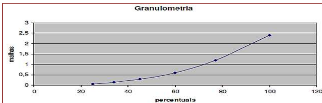
Figura 1: Curva granulométrica do agregado miúdo.
