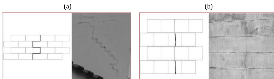
Figura 1- fissuras desenvolvidas pela tração dos materiais
