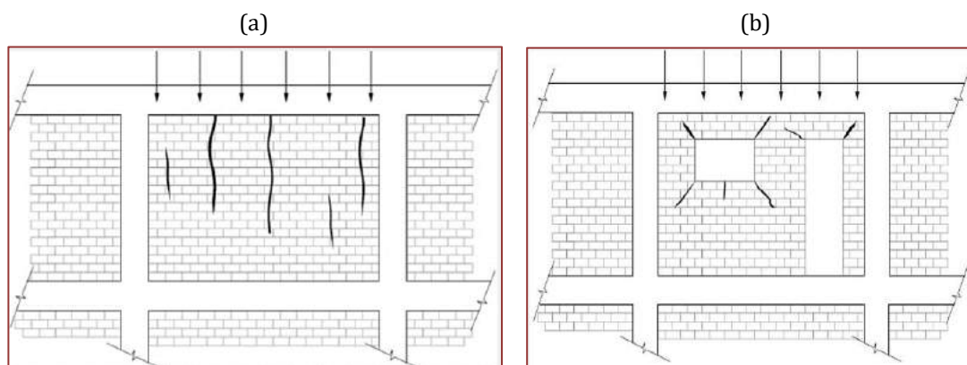
Figura 2- trincas, fissuras e rachaduras causadas pela ação das forças solicitantes
