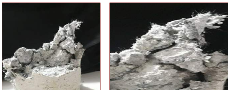
Figura 8: Corpo de prova com adição da FP rompido aos 28 dias
