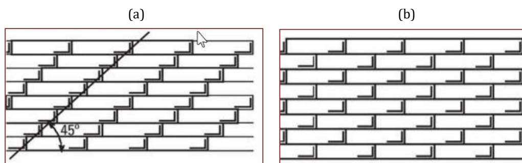
Figura 5- Combinações do uso de tijolos na alvenaria
