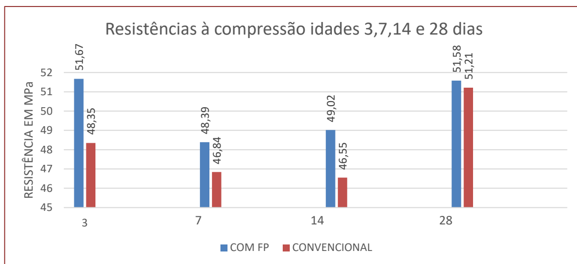
Figura 6: Comparação entre as resistências à compressão média do concreto com fibra e sem fibra das idades 3, 7, 14 e 28 dias.
