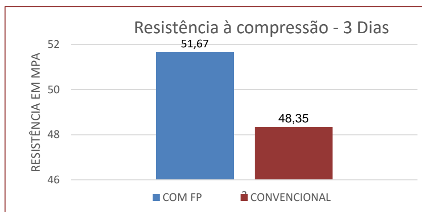
Figura 2: Resistência à compressão média do concreto com fibra e sem fibra com idade de 3 dias.
