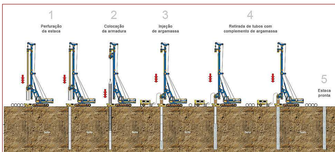
Figura 2: Estaca escavada.
