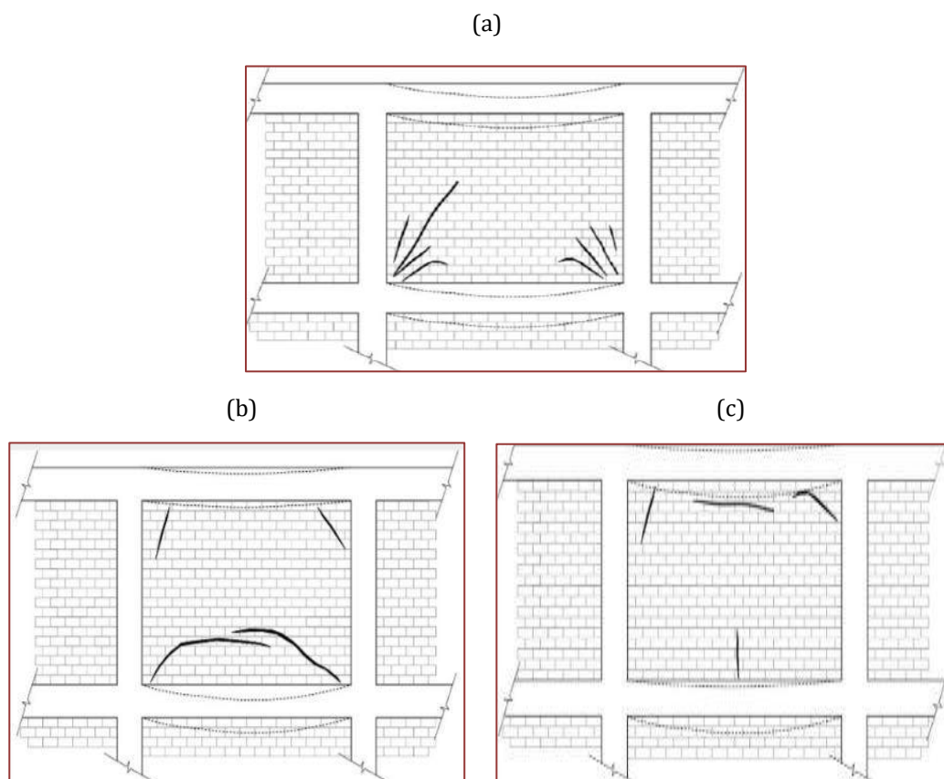
Figura 3- fissuras, trincas e rachaduras por deformações
