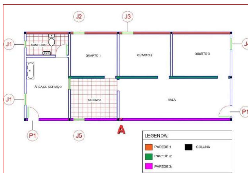
Figura 3 - Planta baixa
