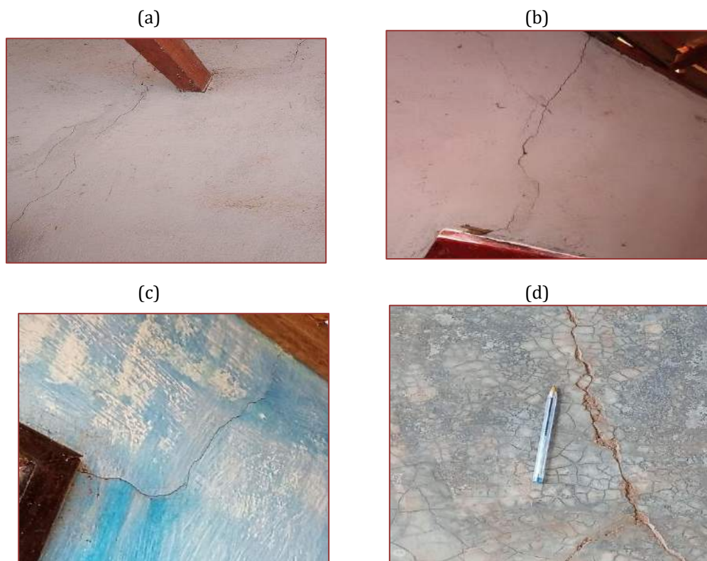
Figura 1- fissuras, trincas e rachaduras do Caso1.
