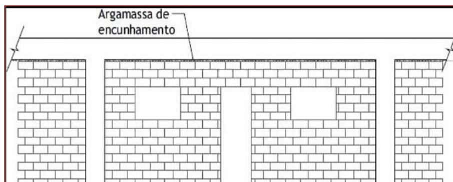
Figura 4- exemplo de alvenaria bem executada
