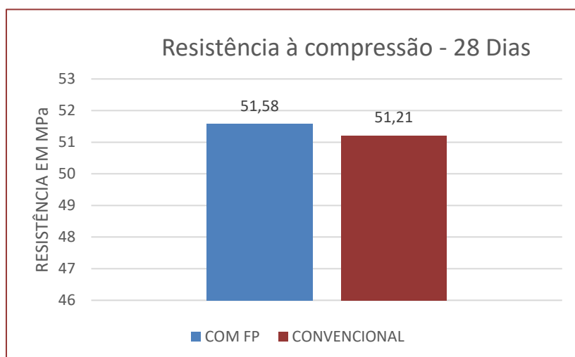
Figura 5: Resistência à compressão média do concreto com fibra e sem fibra com idade de 28 dias.
